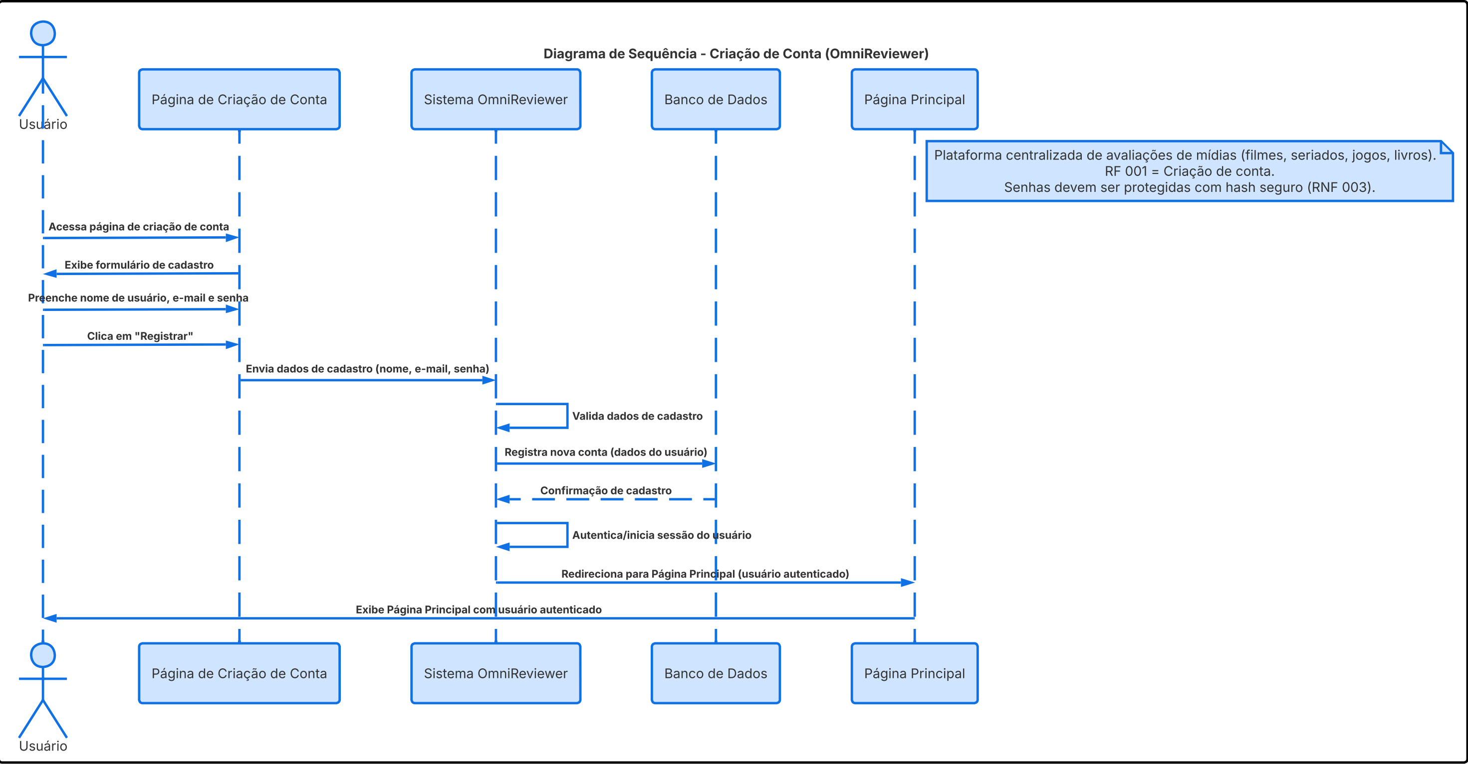
Diagrama de Sequência - Criação de Conta (OmniReviewer)
